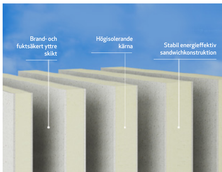
Närbild av Zenergys ZIP-element
