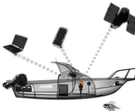
Installerad C-Pod i en motorbåt som kommunicerar via GSM och GPS.
